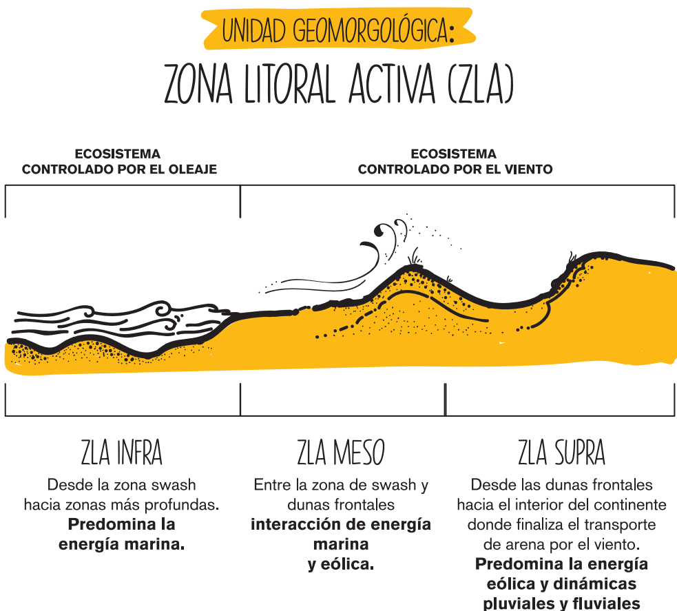
Figura 3: Unidad geomorfológica que se llama “Zona Litoral Activa” (ZLA).
