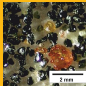
Figura 1: Diferentes tipo de arena, su color y tamaño del grano vistas al microscopio.
